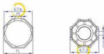
DH29 Corona DL32 Adattatore
