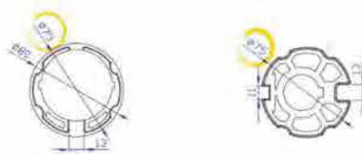
DH54 Corona DL64 Adattatore
