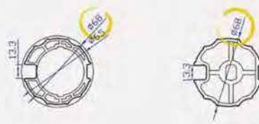
DH142 Corona DL160 Adattatore
